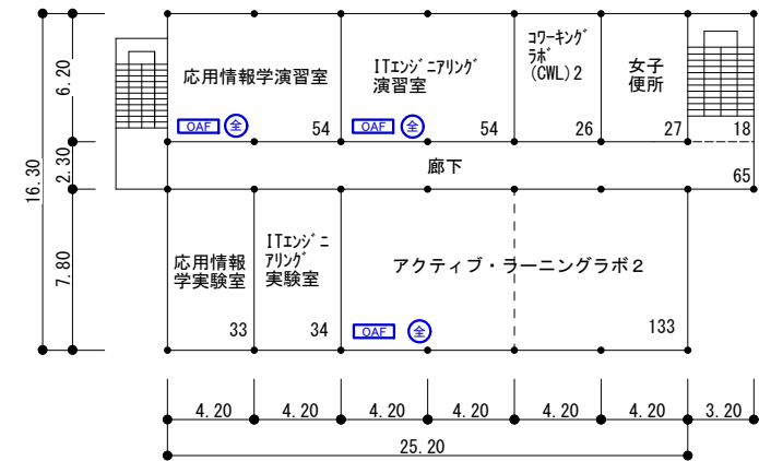
(改修後)流通情報工学科校舎3階平面図 1/400
