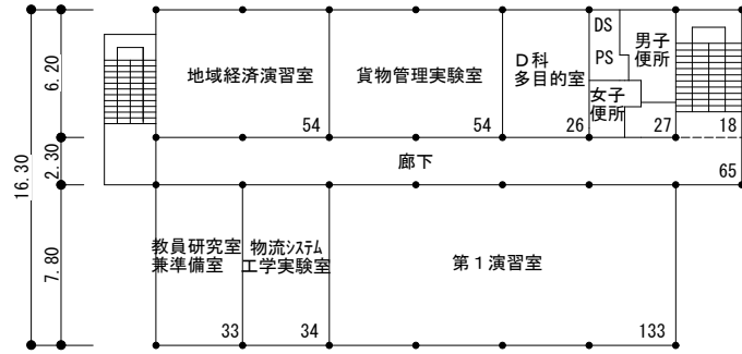
(改修前)流通情報工学科校舎2階平面図 1/400
