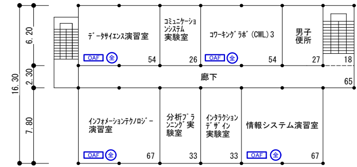
(改修後)流通情報工学科校舎4階平面図 1/400
