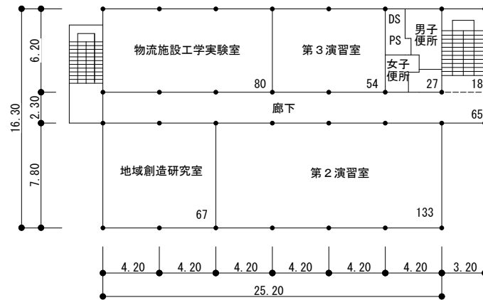
(改修前)流通情報工学科校舎3階平面図 1/400
