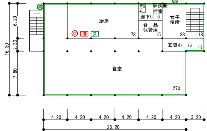
(改修後)流通情報工学科校舎1階平面図 1/400
