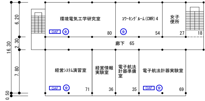
(改修後)流通情報工学科校舎5階平面図 1/400
