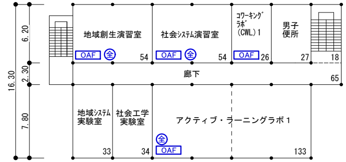
(改修後)流通情報工学科校舎2階平面図 1/400
