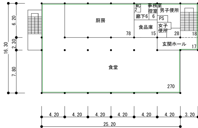
(改修前)流通情報工学科校舎1階平面図 1/400
