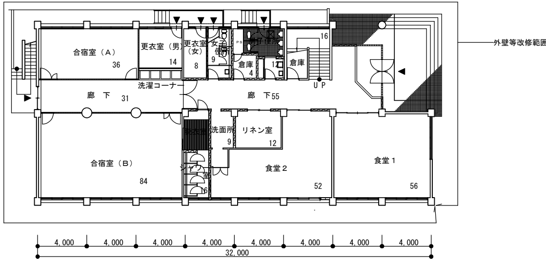
福利施設1階平面図
