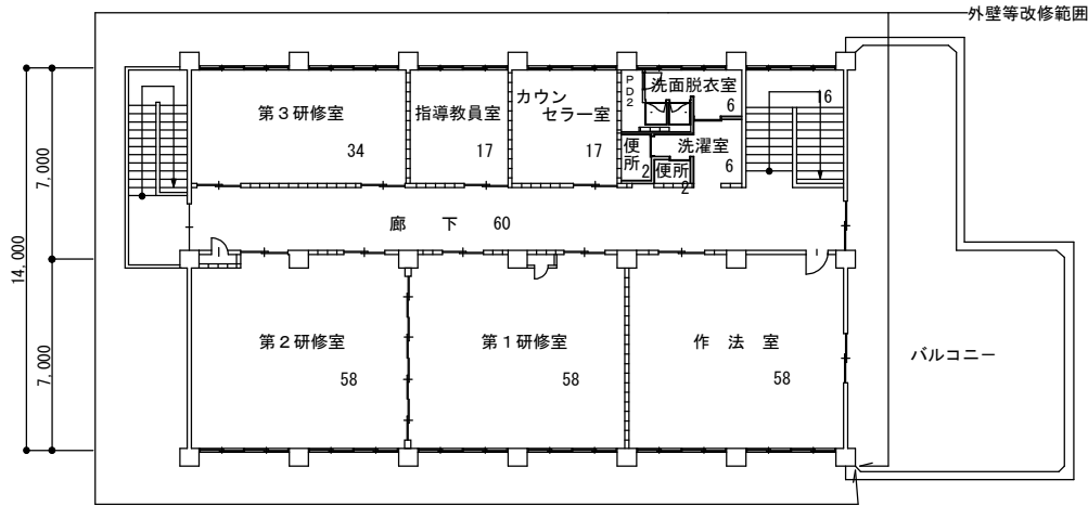
福利施設2階平面図
